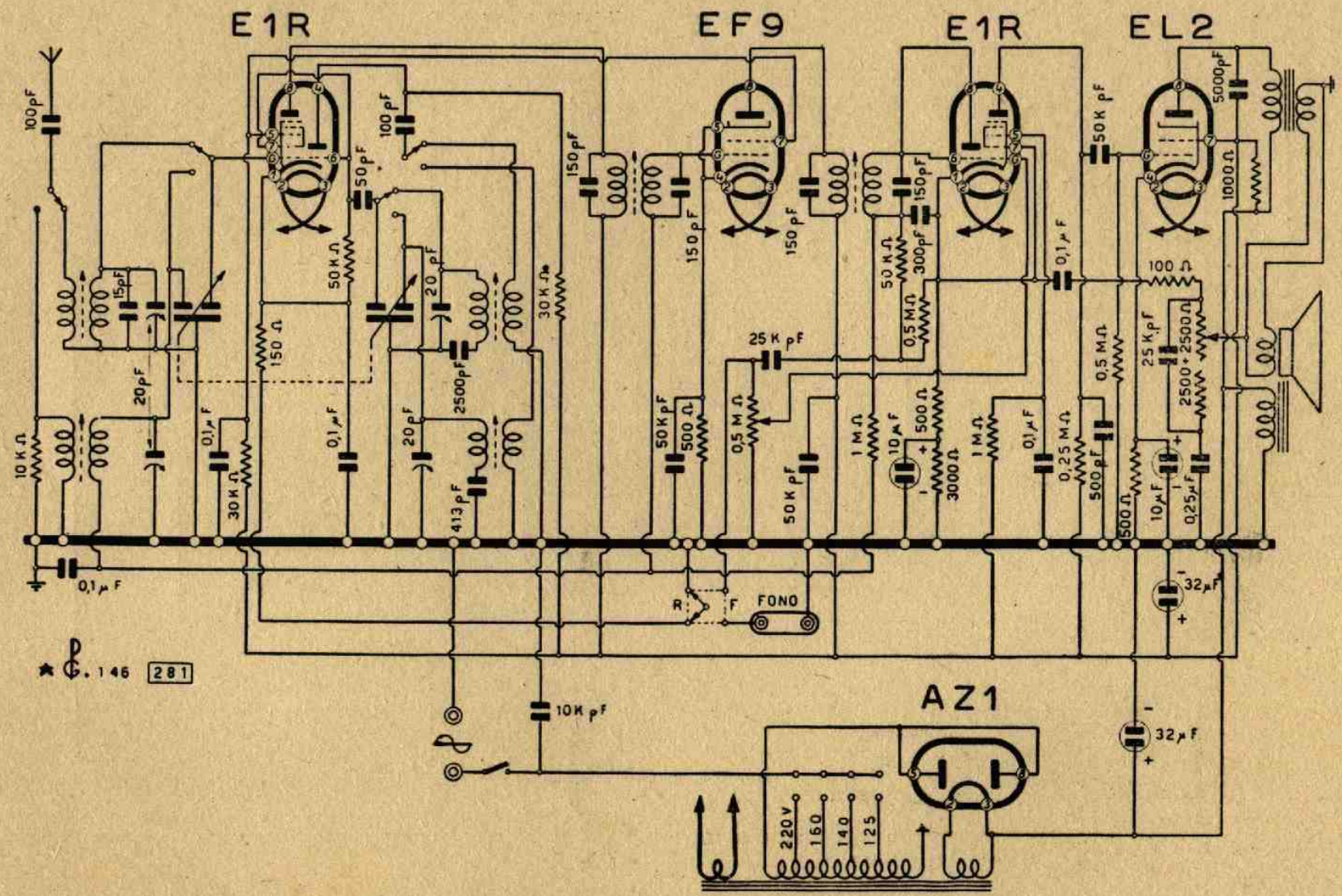
Lo schema elettrico del mod. 525 V (radiofono valigia).
